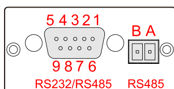
Рис. 2-21 Плата конвертора протоколов
