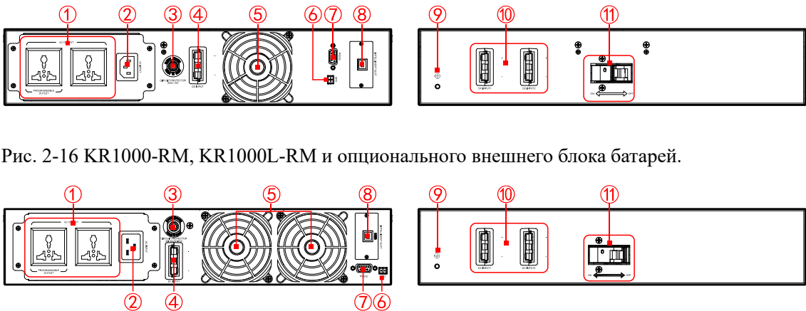
Рис. 2-17 Задняя панель KR2000-RM / KR3000-RM, KR2000L-RM / KR3000L-RM и опционального внешнего блока батарей.
