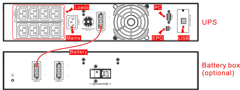
Рис. 3-2 Схема подключения KR1000-RM/KR1000L-RM
